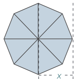
TEATRO PRO Ø250 X=1350 MM
